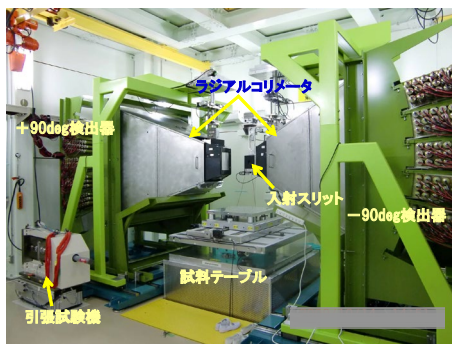
J-Parc MLF : BL19工学回折装置「匠」、BL03生命物質構造解析装置iBIX
